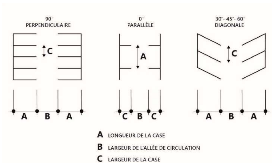
Figure 8 - Démonstration des dimensions des cases de stationnement
