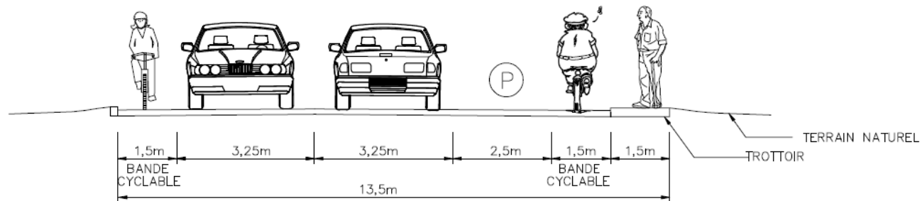
Figure 12 Coupe type proposée pour le chemin d'Old Chelsea - immédiatement à l'est du chemin Scott
