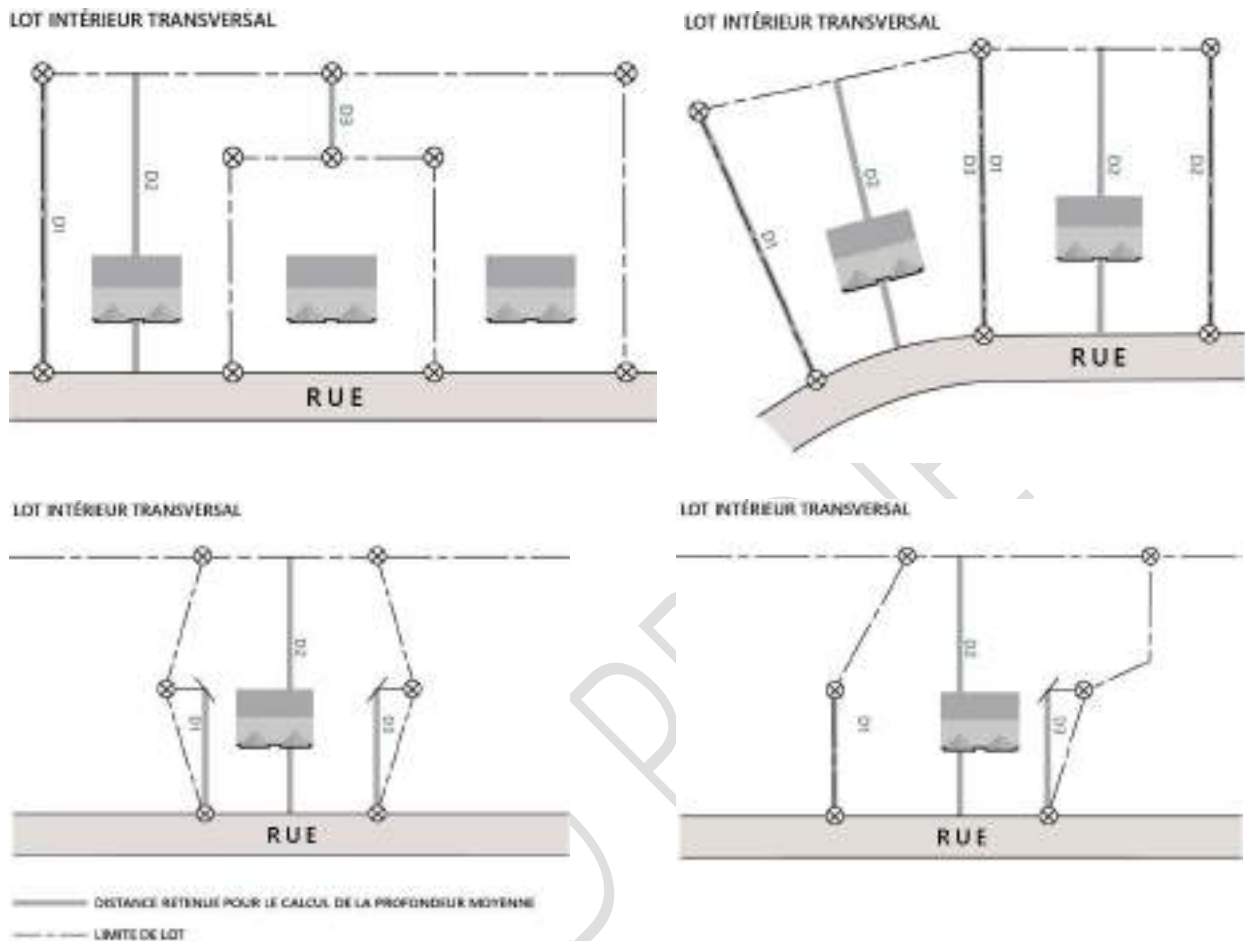
Figure 7 - Calcul de la profondeur minimale d'un lot
