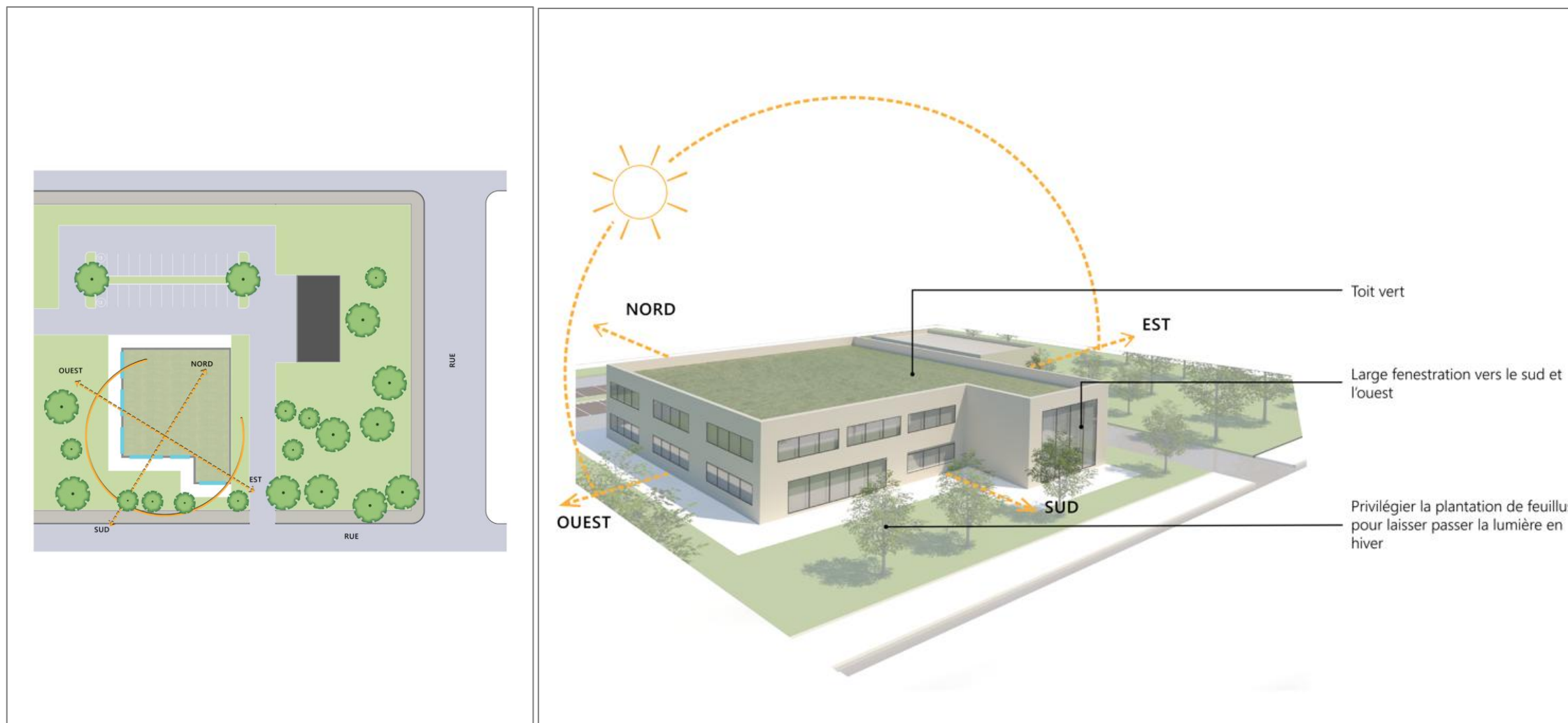
Figure 6 - Les bâtiments sont largement fenestrés sur les façades orientées au sud et non exposées aux vents dominants.
