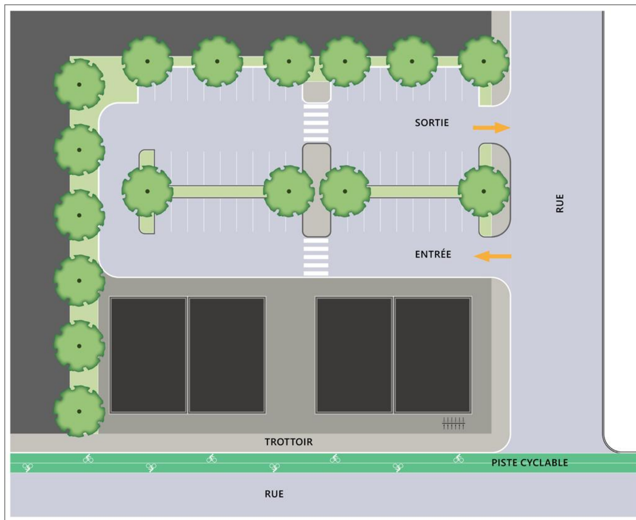
Figure 9 - Les entrées et sorties sont bien délimitées par des entrées charretières, accompagnées d'indications précises et aménagées avec divers éléments de végétation.
