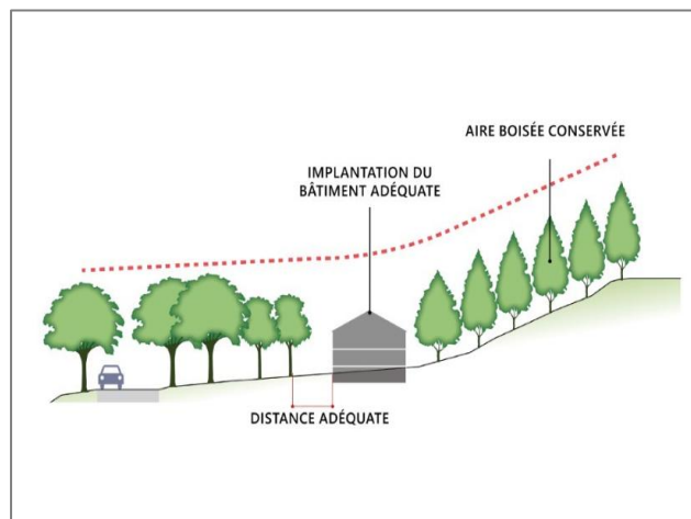
Figure 4 - L'implantation des bâtiments s'adapte à la topographie naturelle du terrain afin de sauvegarder le plus possible la végétation existante et restreindre au minimum les déblais et remblais autour du bâtiment.
